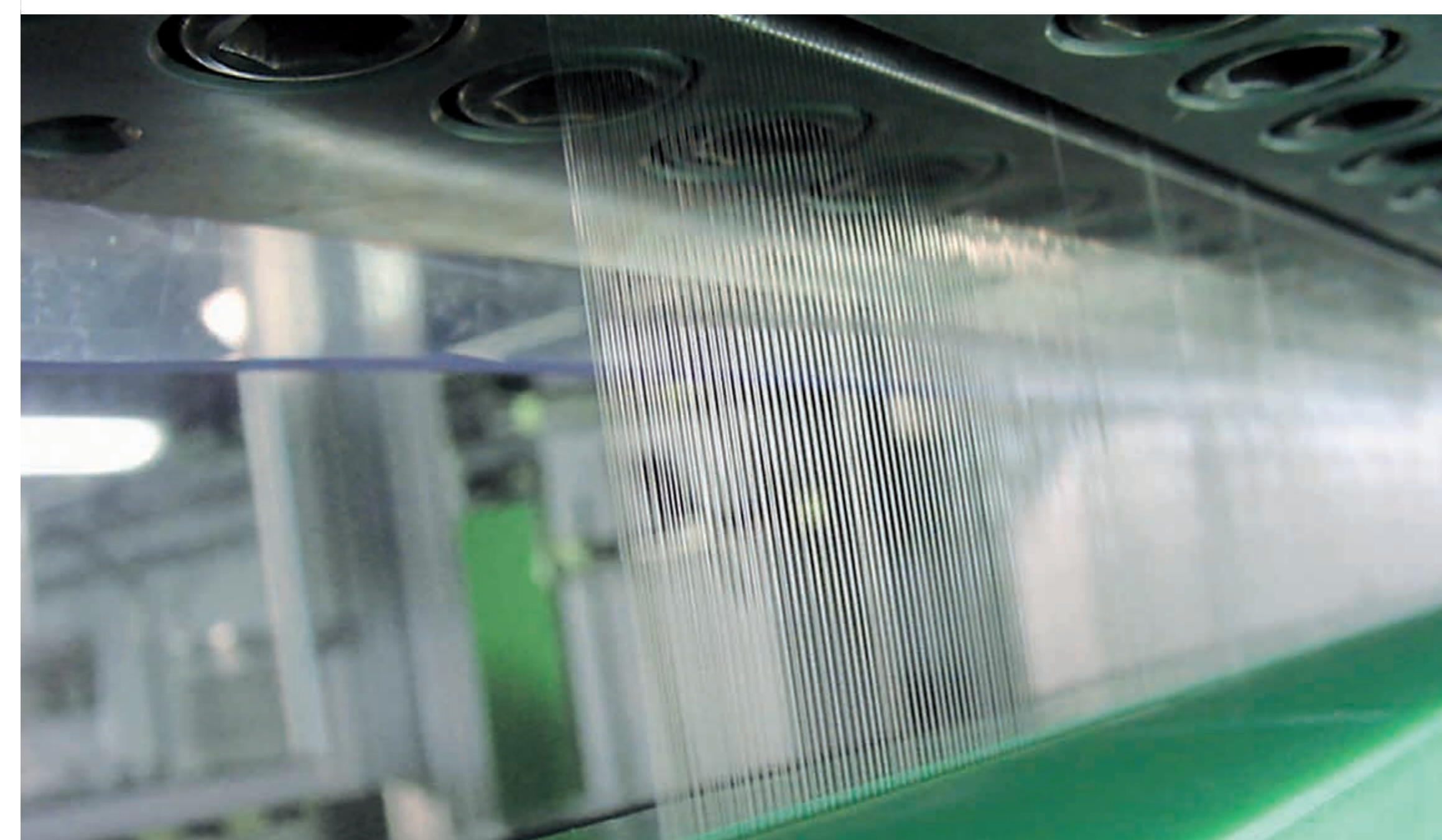
Spunlace Line
